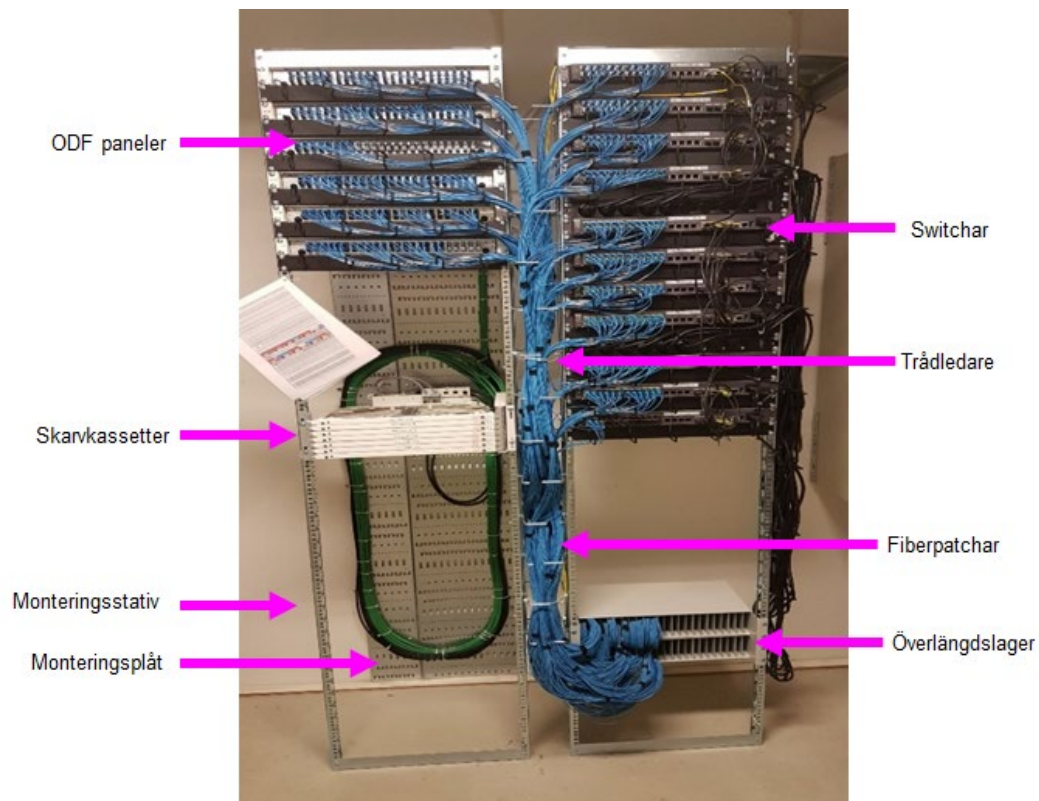
Bild ODF-stativ med installerade switchar
