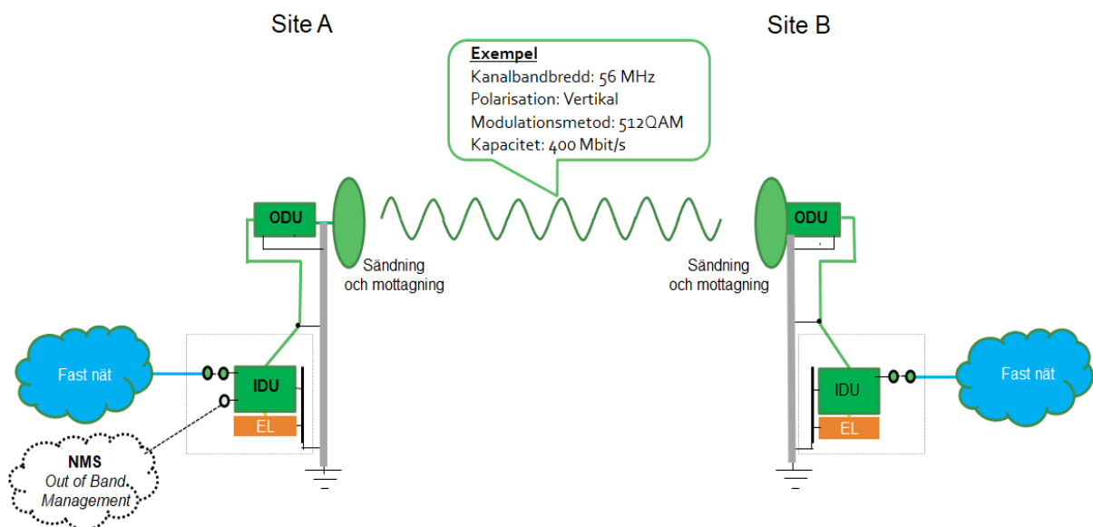
Bild 1. Grundkonfiguration (1+0) radiolänk
