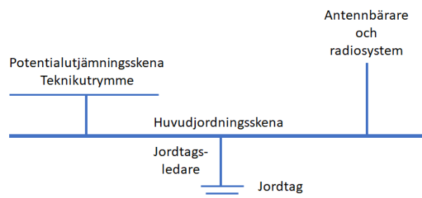
Bild 13. Jordsystem
